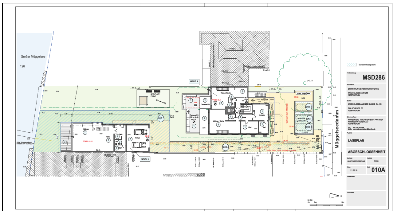
Lageplan
