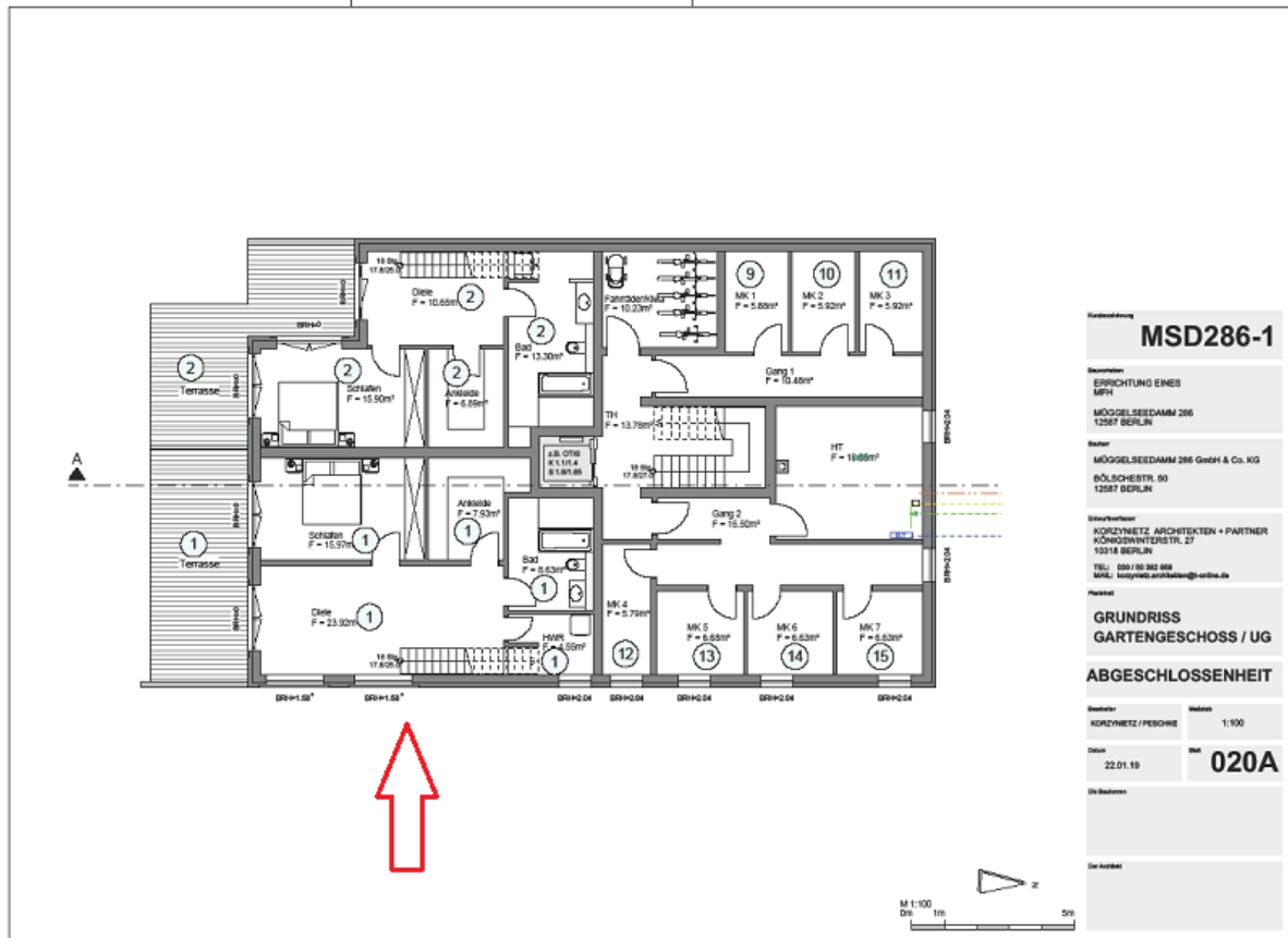
Gartengeschob
