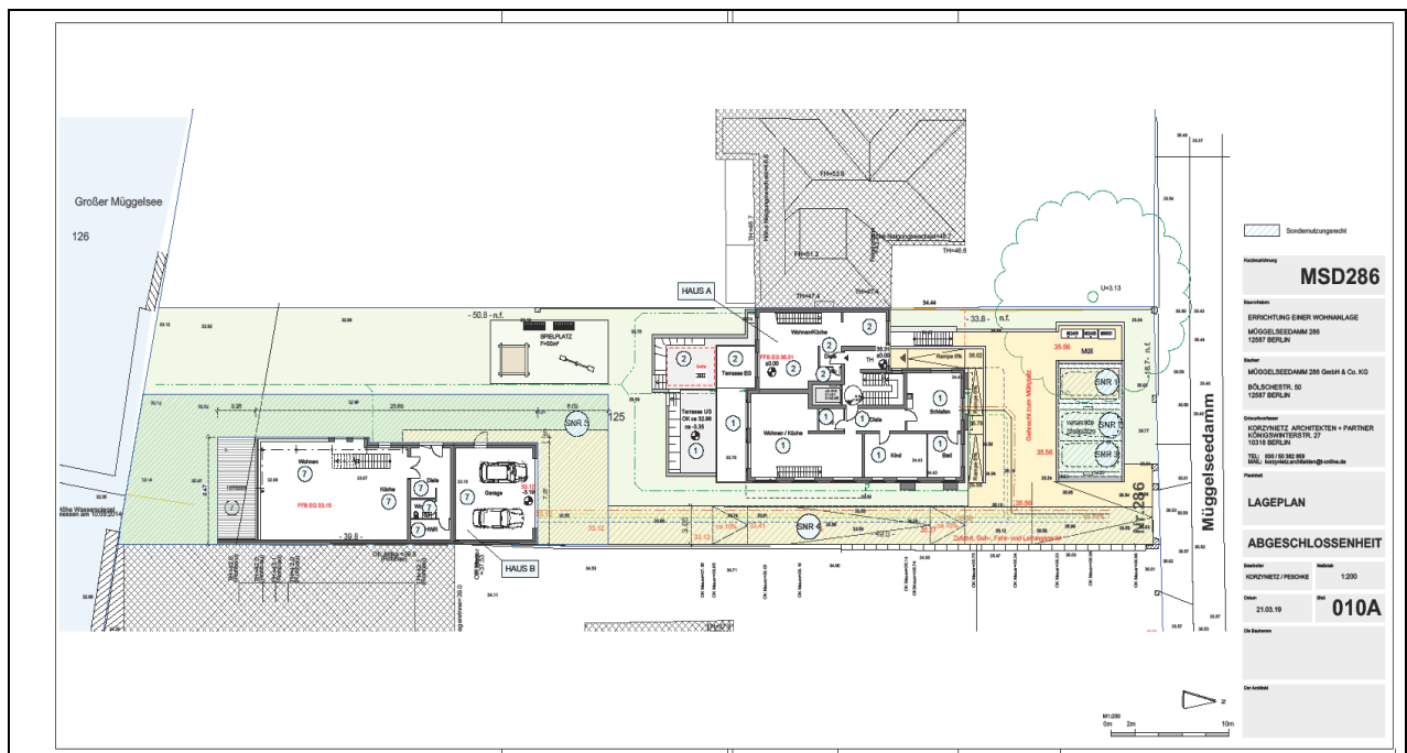
Lageplan
